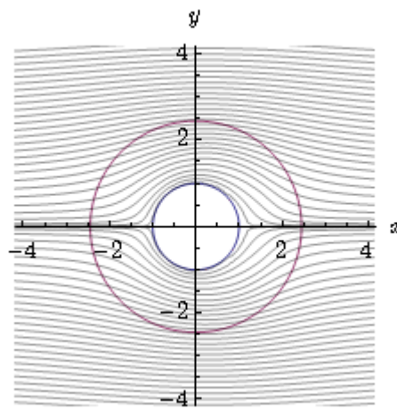
Рис. 2. Линии уровня функции тока при Re = 5
